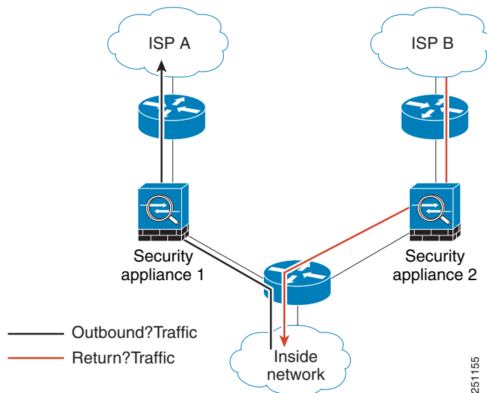
图 12-1 非对称路由：
