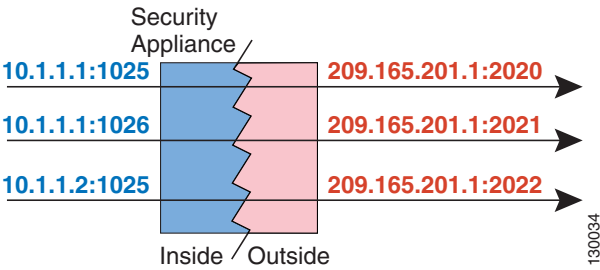
图 4-10 动态 PAT
