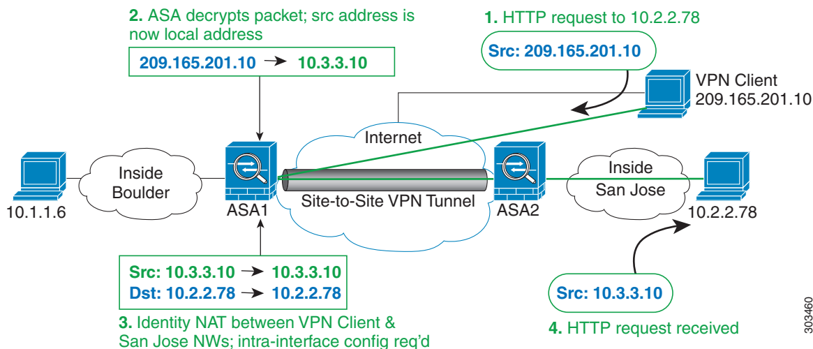
图 4-24 VPN 客户端访问站点到站点 VPN
