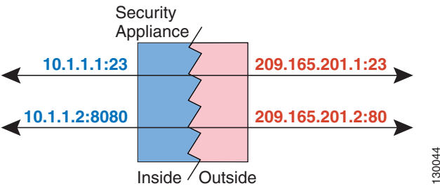
图 4-2 带端口转换的典型静态 NAT 场景
